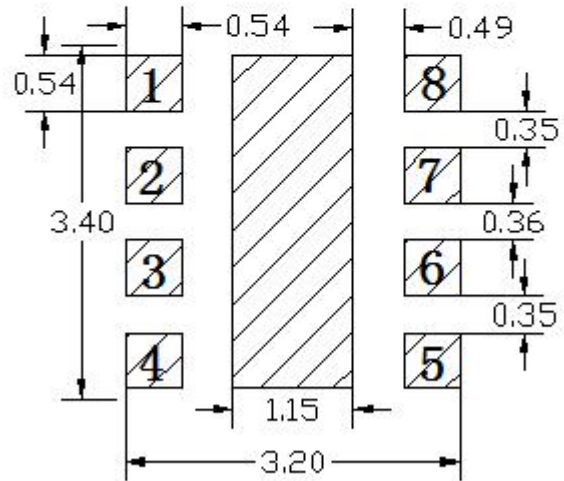
建议焊盘
