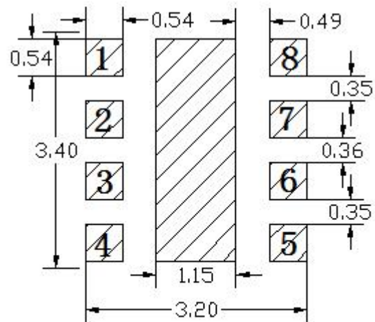
建议焊盘
